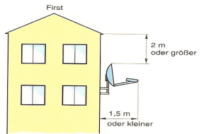
Schutzbereich des Hauses Grafik: Saupe
